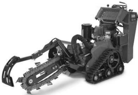
TORO SLEUVENFREES/KETTINGGRAVER
