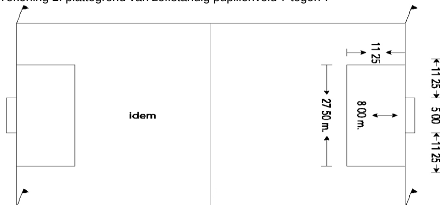
Tekening 2: plattegrond van zelfstandig pupillenveld 7 tegen 7
