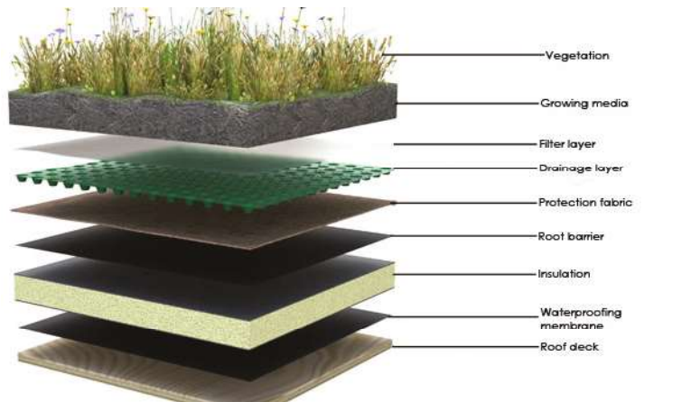
Een vegetatiedak biedt vele voordelen; dak gaat langer mee, werkt isolerend, bijdrage aan biodiversiteit, kan in combinatie met zonnecellen
